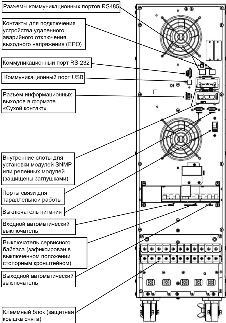
Рисунок 2.2 — Общий вид задней панели изделий SKAT-UPS 15-3/3-ON-2x(20x9) и SKAT-UPS 20-3/3-ON-2x(20x9) со снятой крышкой клеммного блока
